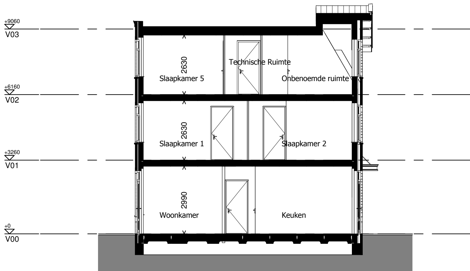
Doorsnede
