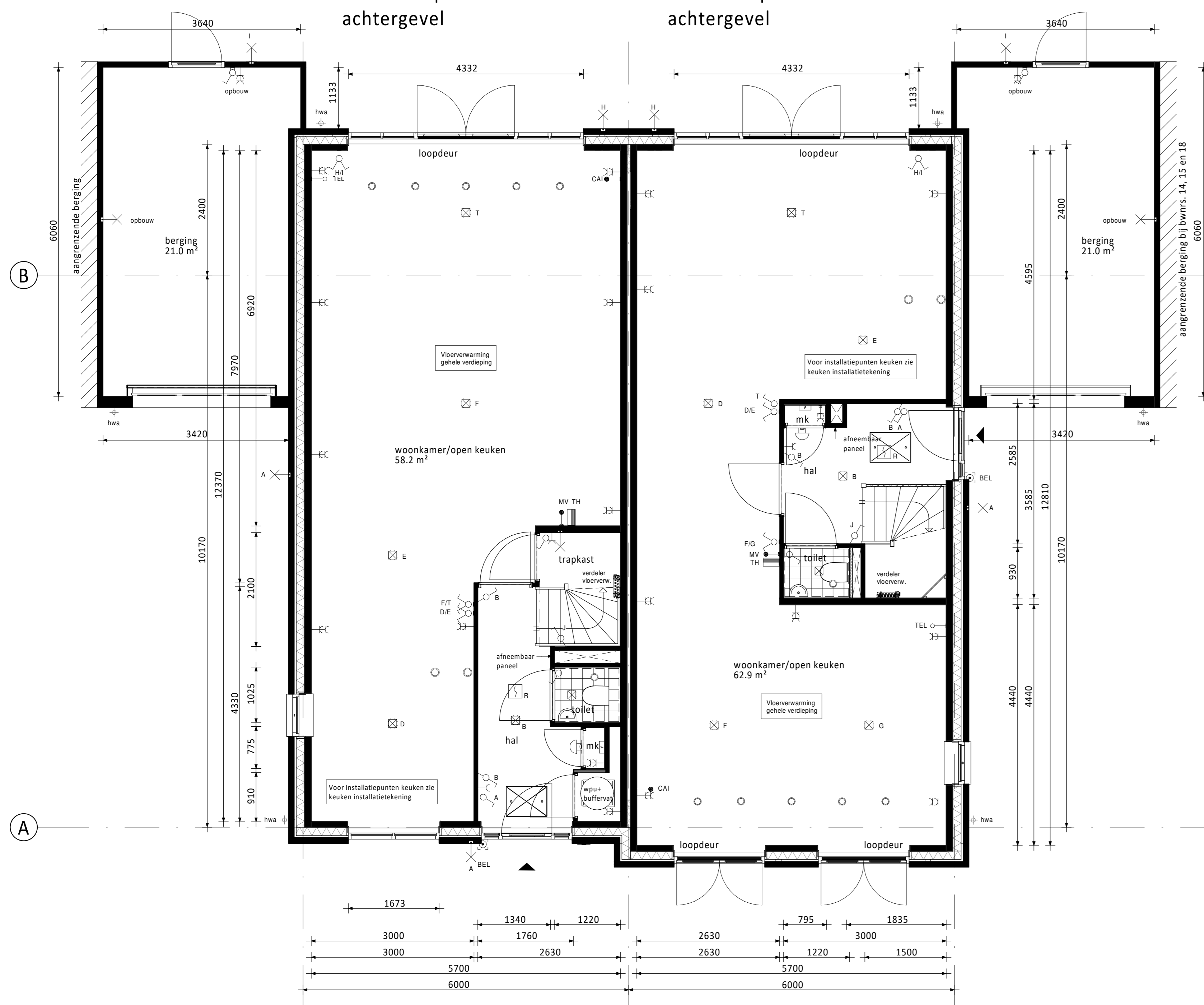
Begane grond ① Type C • Verdiepingshoge pui voorgevel • Aanbouw 2,4m achtergevel (op de begane grond) • Brede gevelpui met dubbele openslaande deuren achtergevel ② Type D • Aanbouw 2,4m achtergevel (op de begane grond) • Brede gevelpui met dubbele openslaande deuren achtergevel
