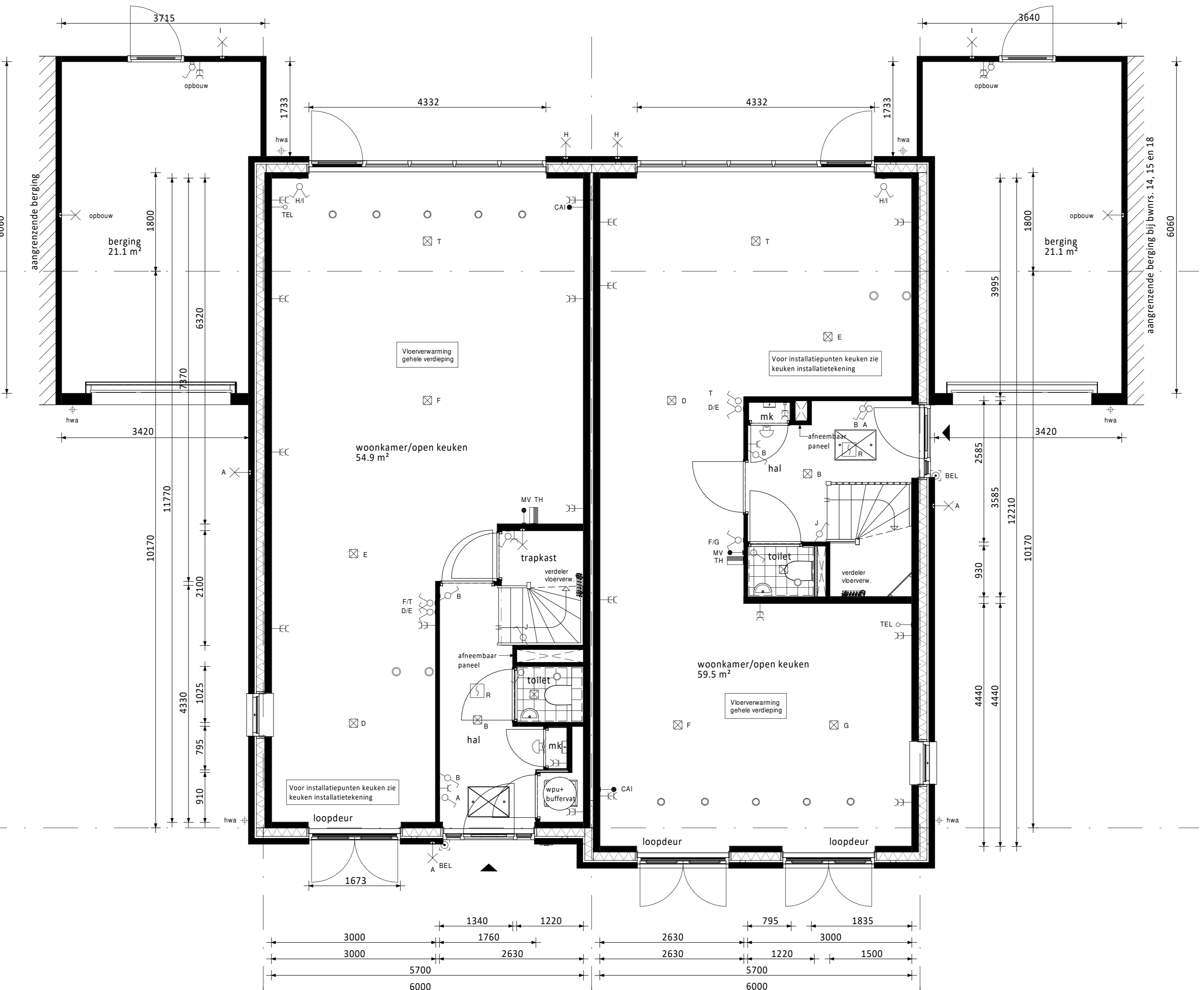
Begane grond ① Type C • Dubbele openslaande deuren voorgevel • Brede gevelpui achtergevel • Aanbouw 1,8m achtergevel (op de begane grond) ② Type D • Brede gevelpui achtergevel • Aanbouw 1,8m achtergevel (op de begane grond)
