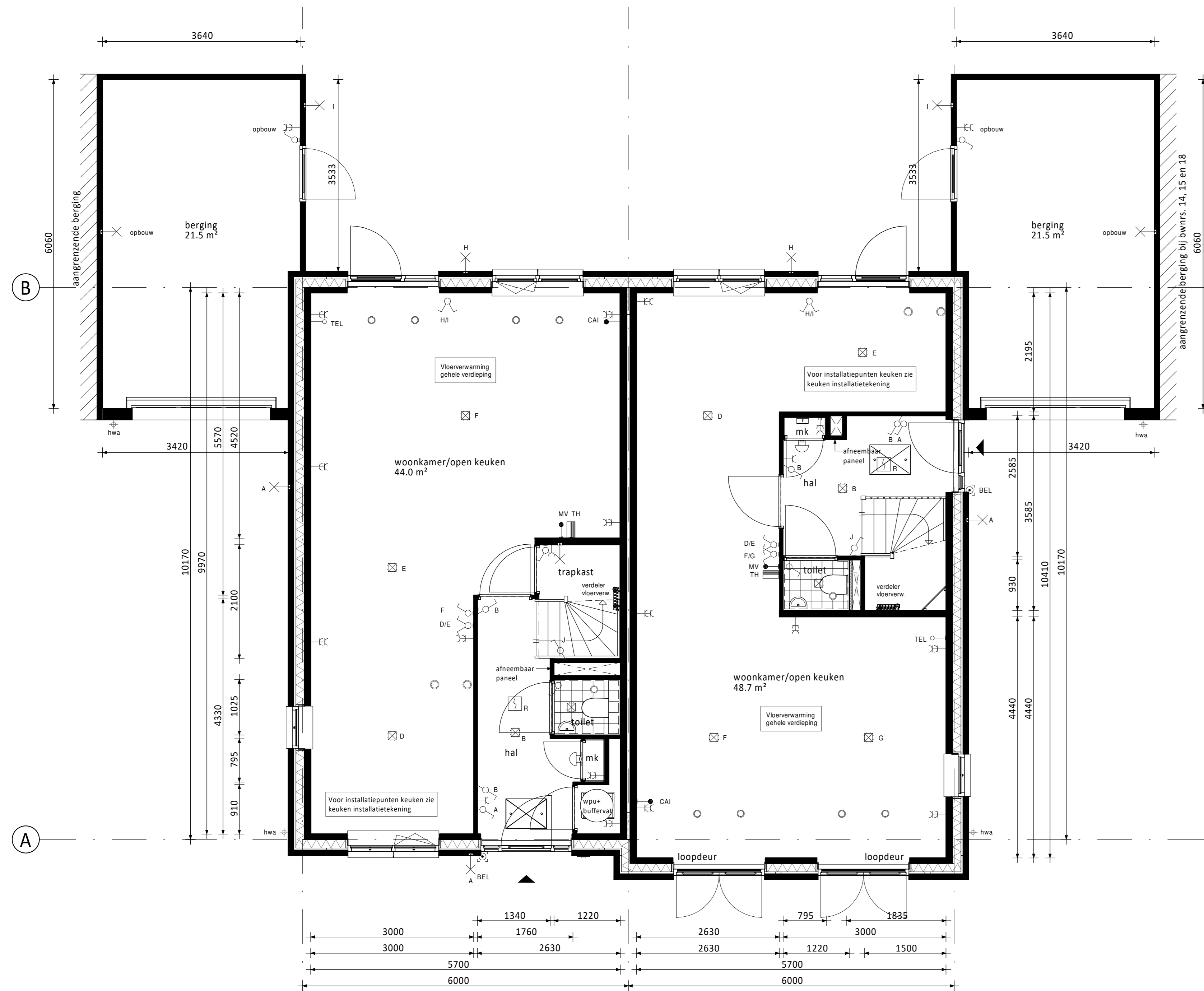
Begane grond ① Type C Bouwnummers 12 en 16 (als getekend) Bouwnummers 13, 17 en 19 (gespiegeld) ② Type D Bouwnummers 11 en 15 (als getekend) Bouwnummers 14, 18 en 20 (gespiegeld)
