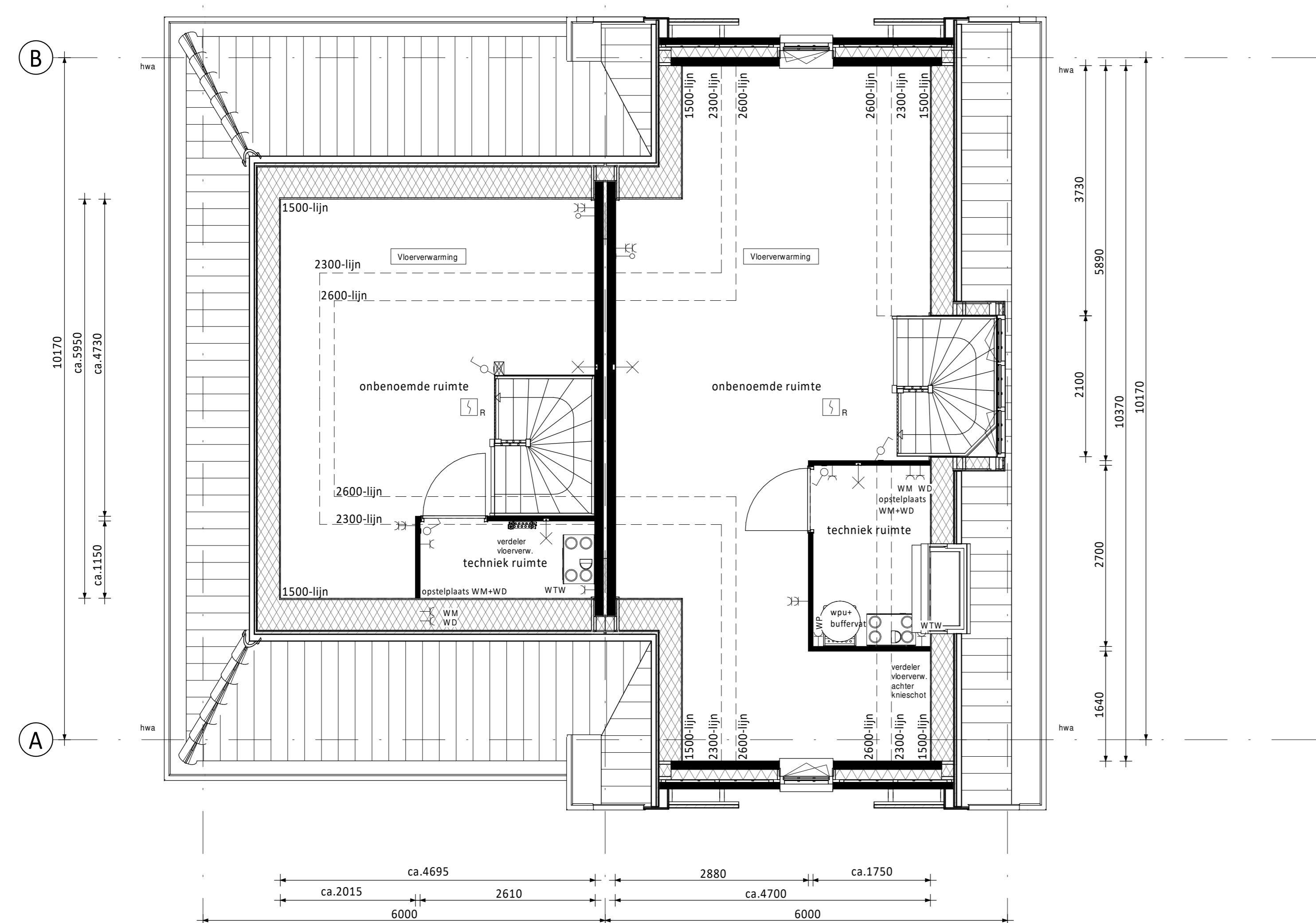
Zolder ① Type C Bouwnummers 12 en 16 (als getekend) Bouwnummers 13, 17 en 19 (gespiegeld) ② Type D Bouwnummers 11 en 15 (als getekend) Bouwnummers 14, 18 en 20 (gespiegeld)
