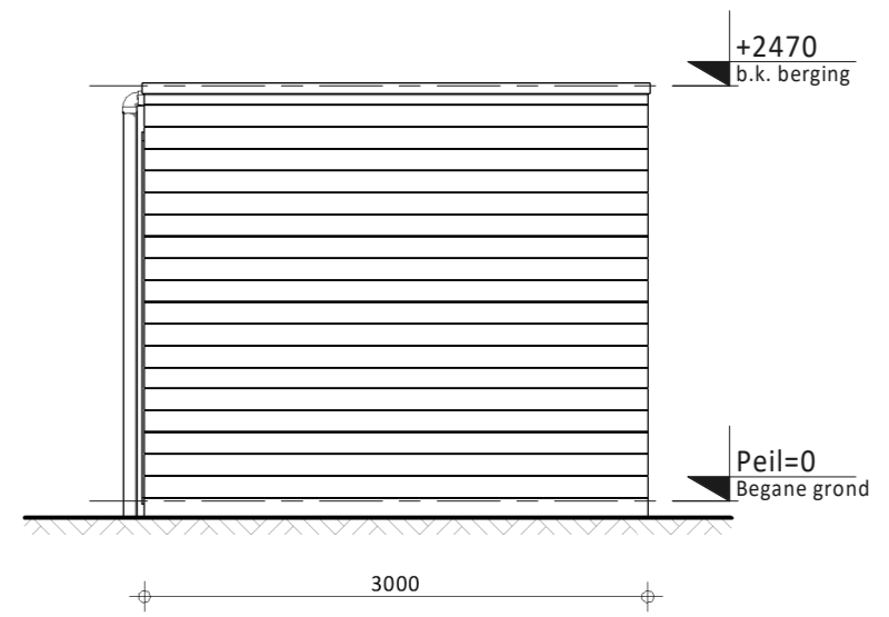
rechter zijaanzicht (type 2)
