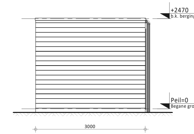
linker zijaanzicht (type 2)
