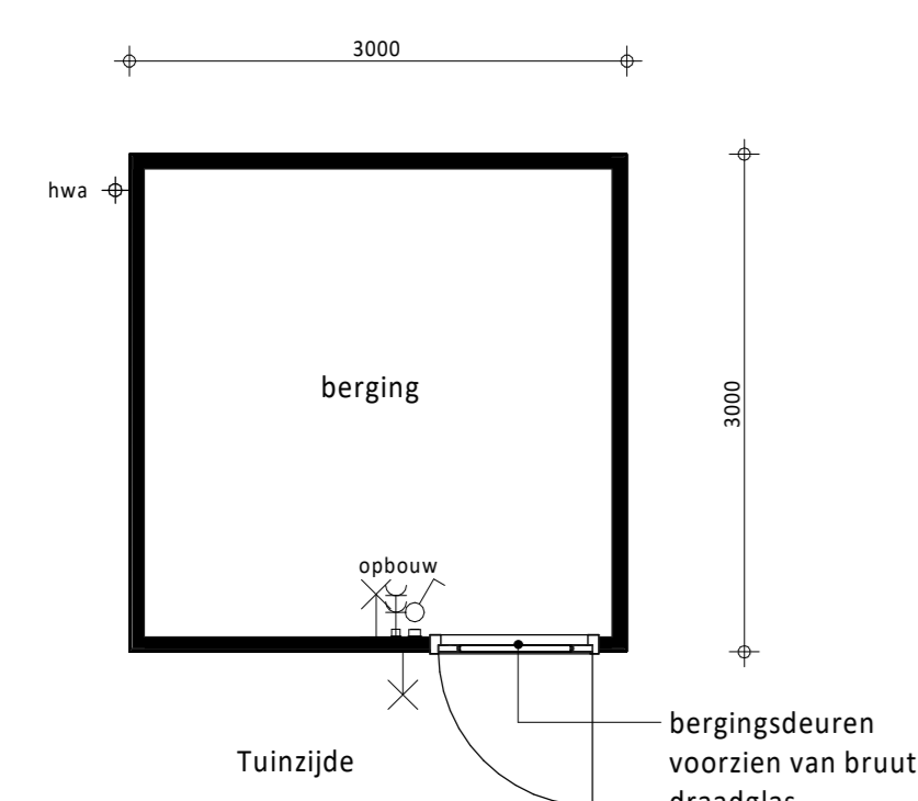
Plattegrond (type 1) 6x uitvoeren bouwnummer getekend: 01, 21, 34 bouwnummer gespiegeld: 10, 33, 41
