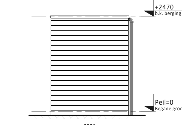
Achteraanzicht (type 3)
