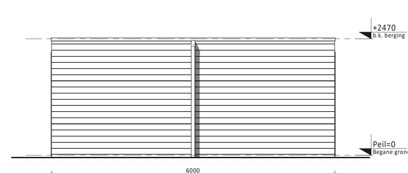
Vooraanzicht (type 4)
