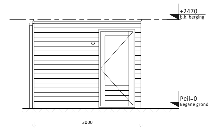
vooraanzicht (type 1)
