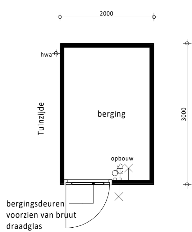
Plattegrond (type 3) 1x uitvoeren bouwnummer: 32
