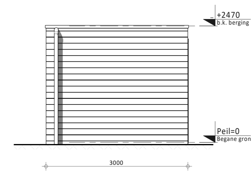
linker zijaanzicht (type 1)
