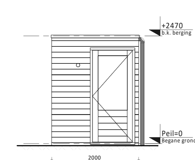
Linker zijaanzicht (type 4)
