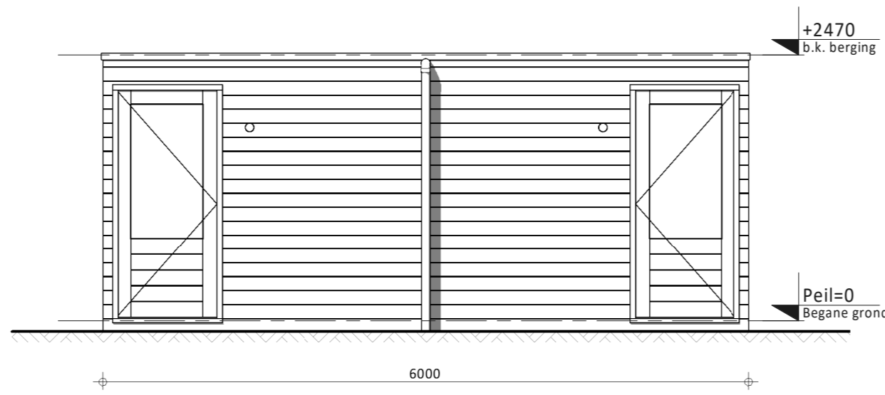
vooraanzicht (type 2)
