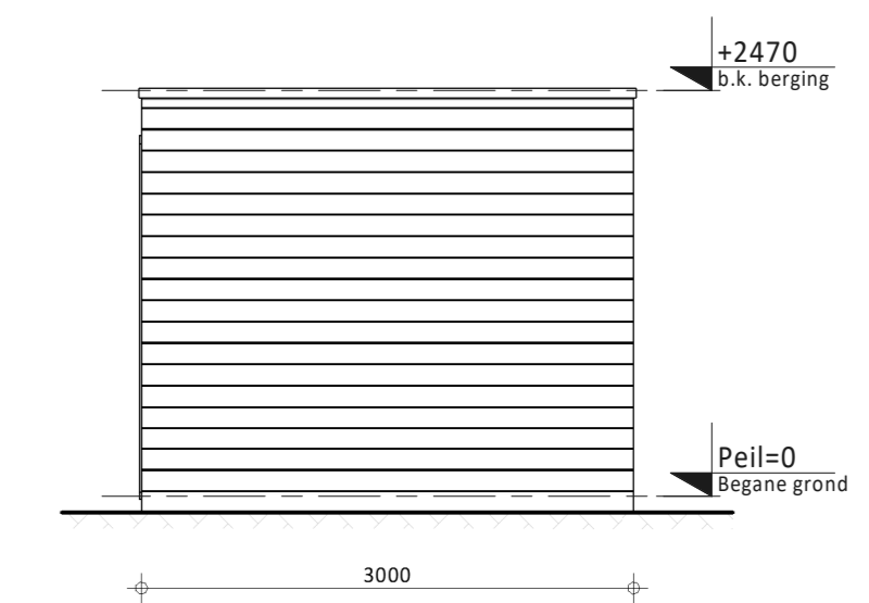
rechter zijaanzicht (type 1)
