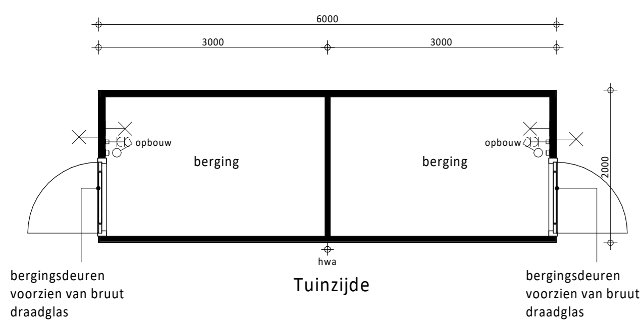
Plattegrond (type 4) 5x uitvoeren bouwnummers: 22/23, 26/27, 30/31, 35/36, 39/40
