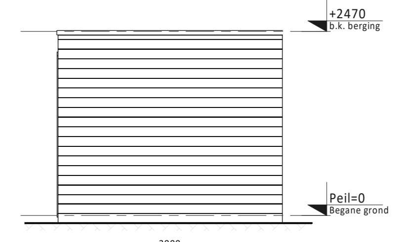
Rechter zijaanzicht (type 3)
