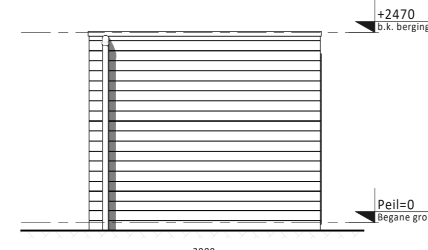
Linker zijaanzicht (type 3)
