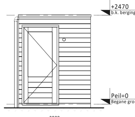
Vooraanzicht (type 3)
