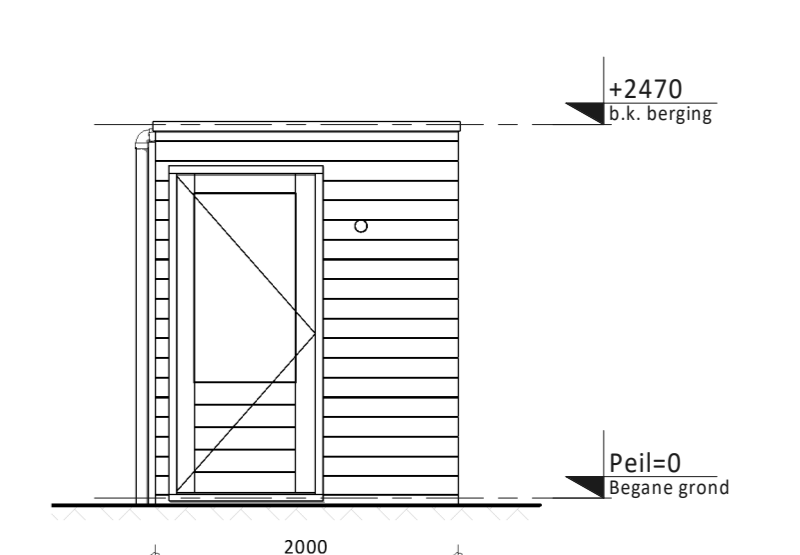
Rechter zijaanzicht (type 4)
