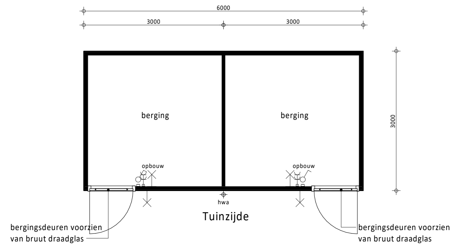
Plattegrond (type 2) 7x uitvoeren bouwnummers: 02/03, 04/05, 06/07, 08/09, 24/25, 28/29, 37/38
